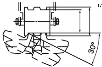
OPTIMALNE PROWADZENIE GĄSIENIC
